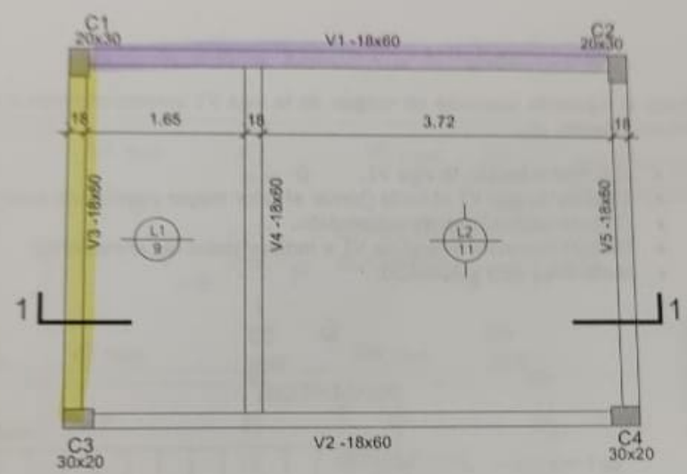
ESTRUCTURA TIPO
