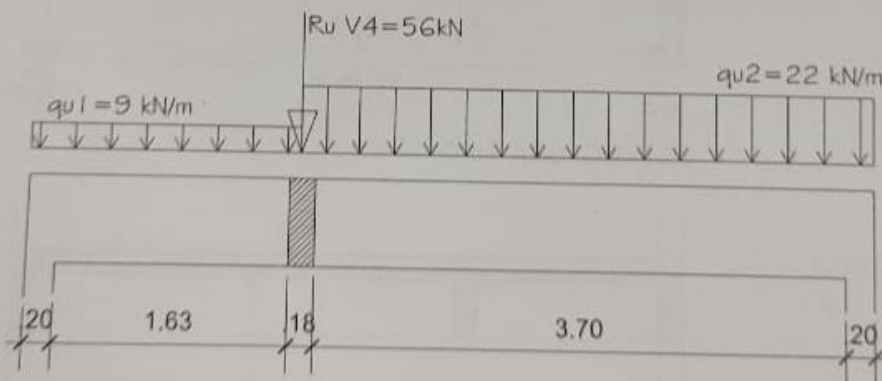
ESQUEMA DE CARGAS V1
