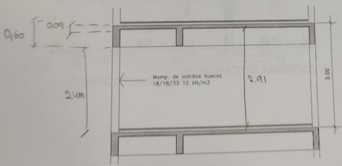
CORTE TRANSVERSAL I-I
